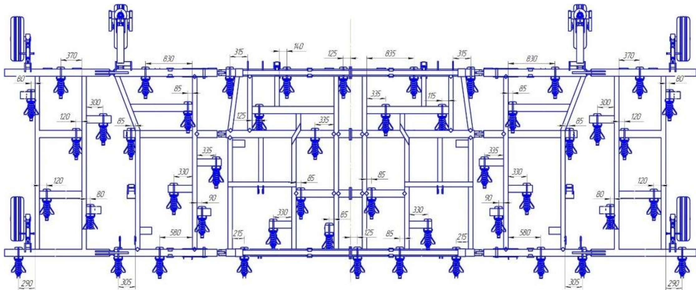
Схема расстановки лапы 355 КРГ-12,0
