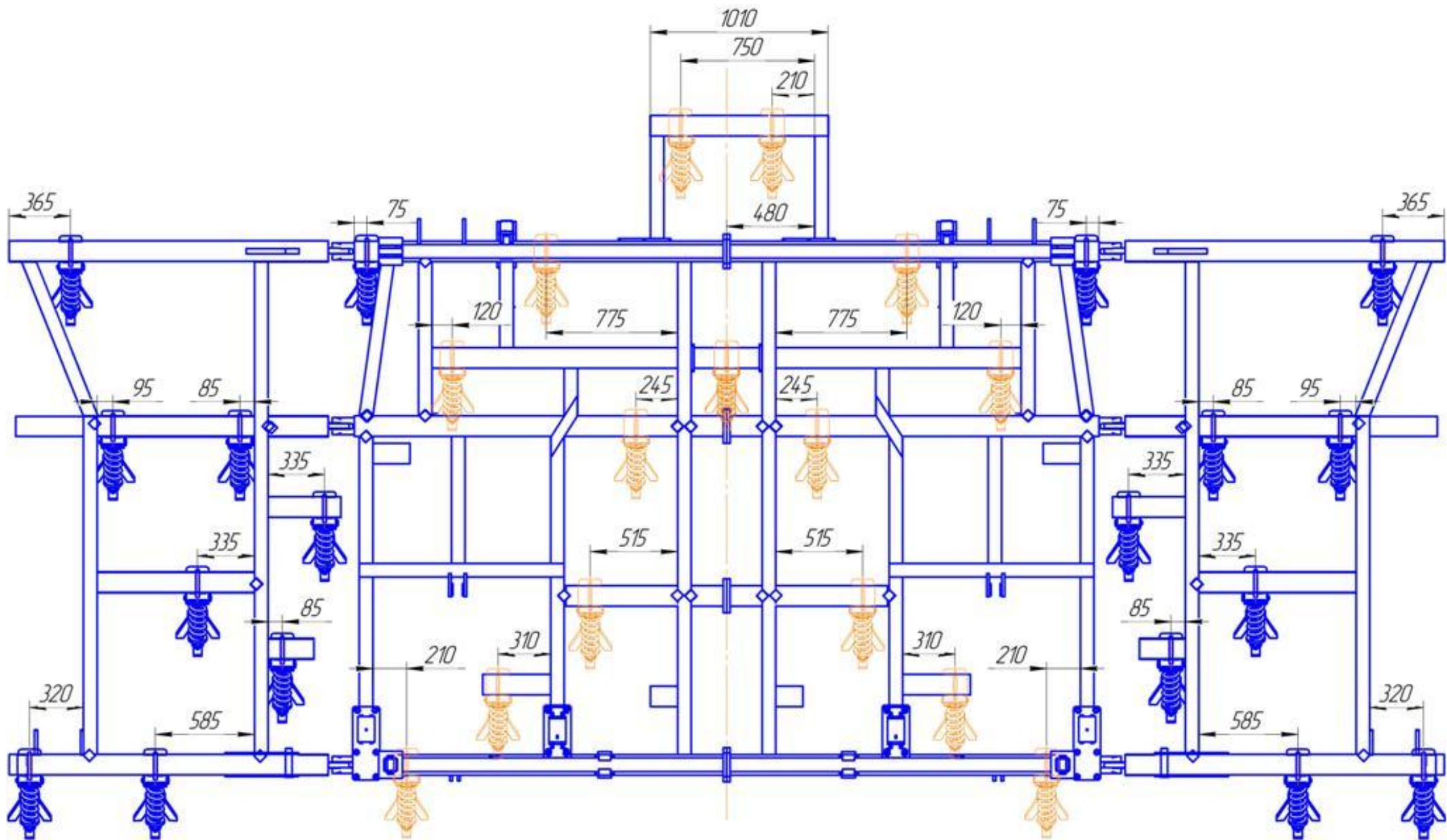
Расстановка КРГ-8,6 лапы 355
