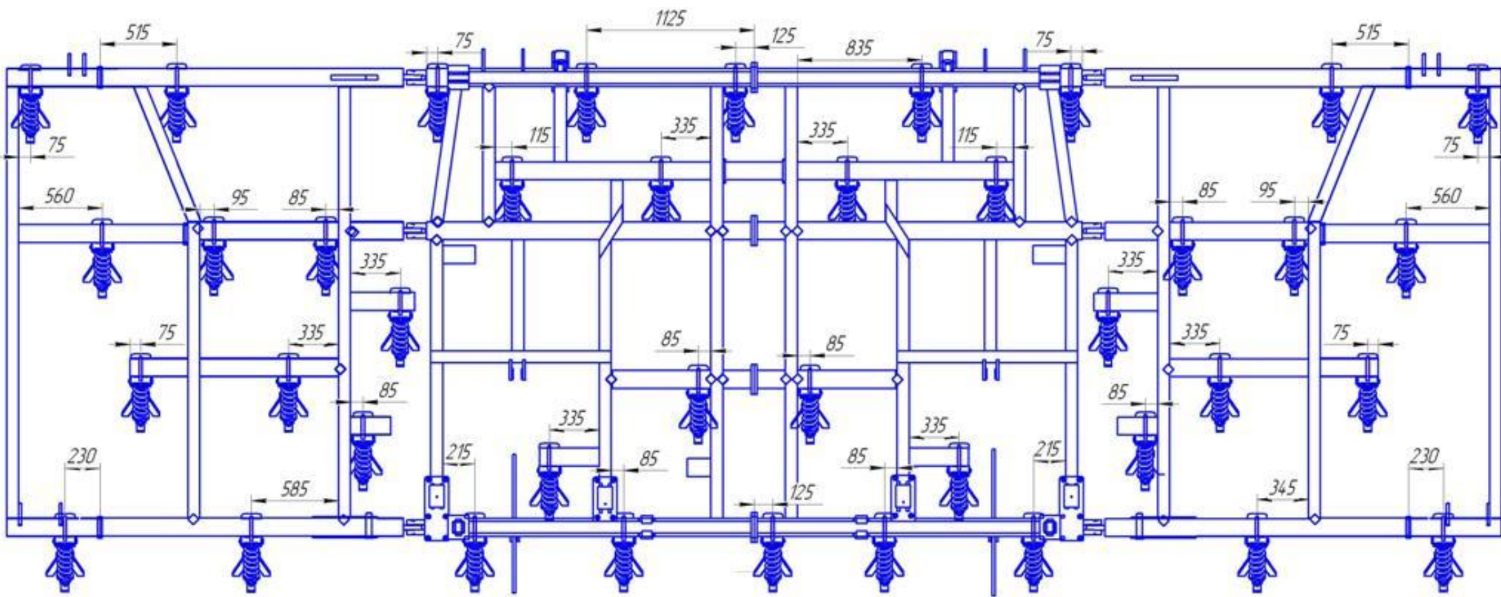
Расстановка КРГ-10 лапы 355
