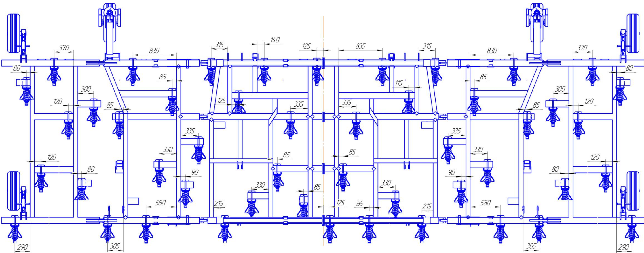
Схема расстановки лапы 355
