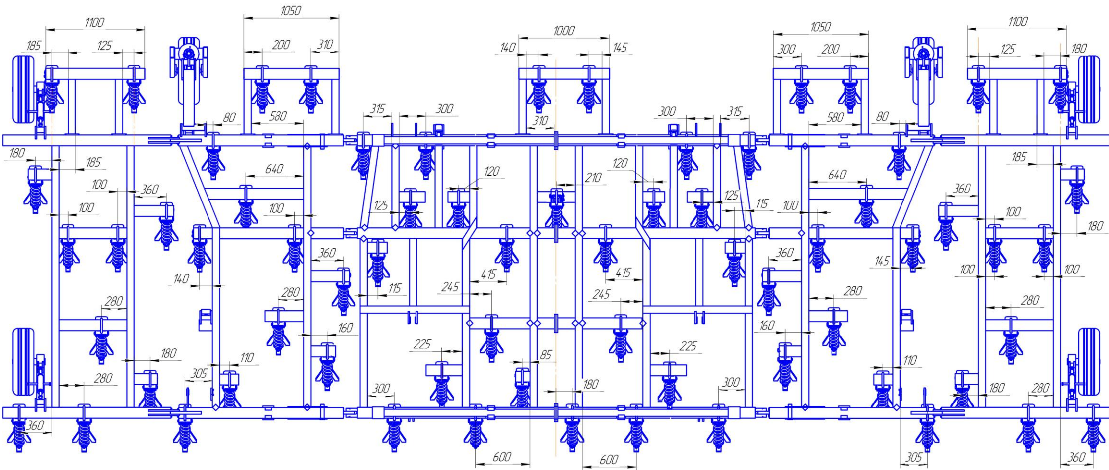
Схема расстановки лапы 255
