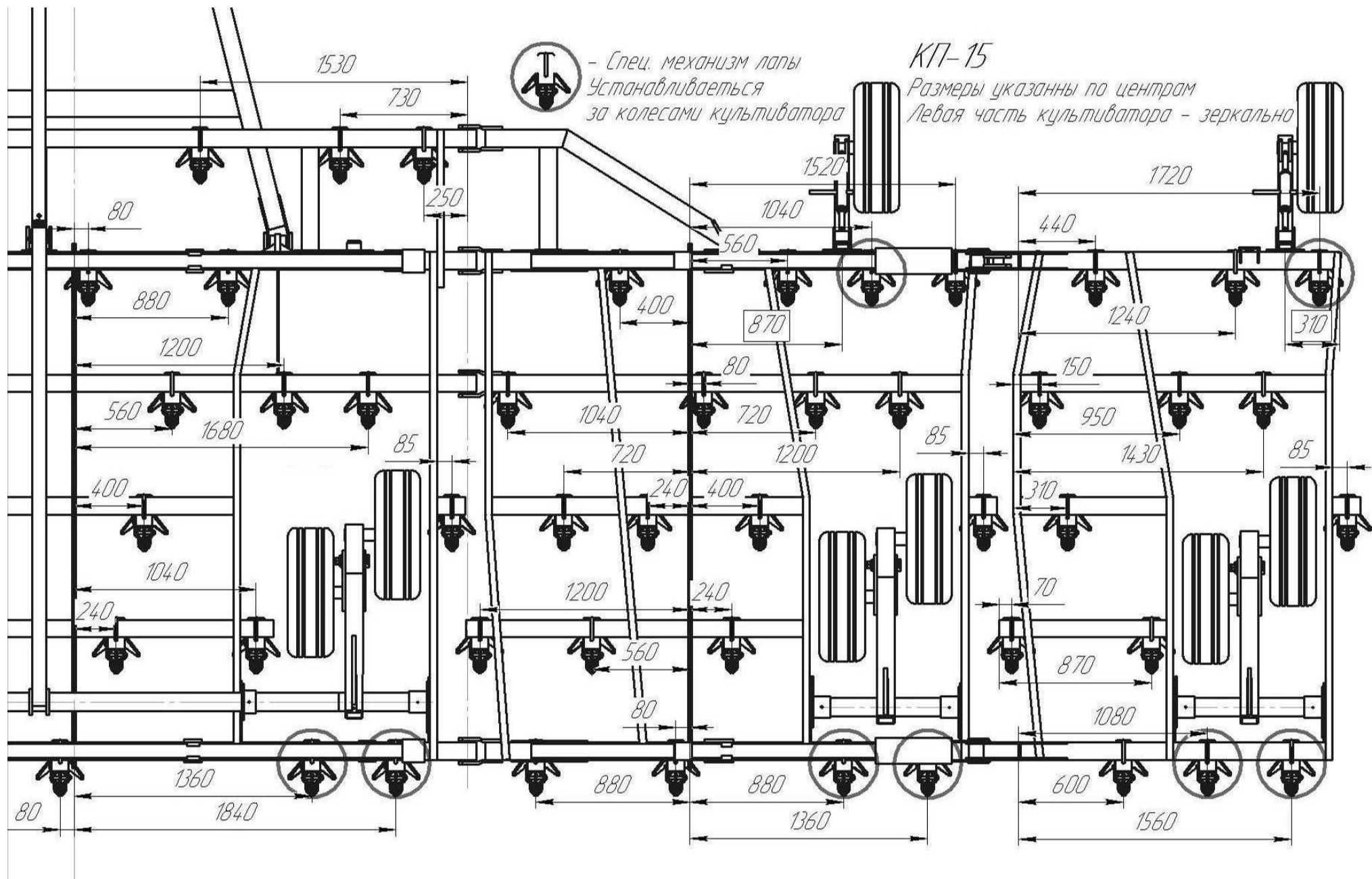
Расстановка механизмов лап КП-15.
