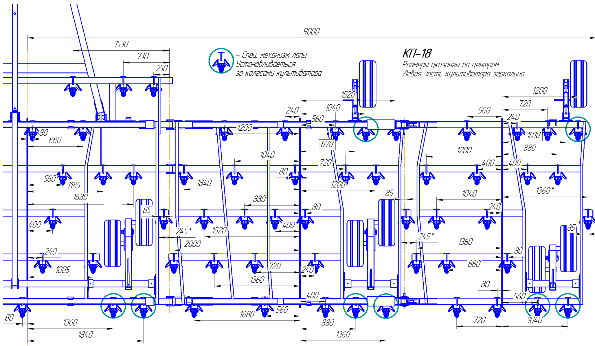
Расстановка механизмов лап КП-18.
